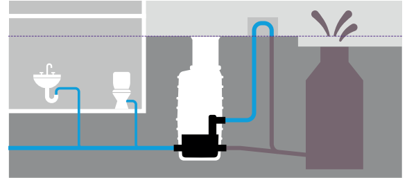
Betrieb bei Rückstau
